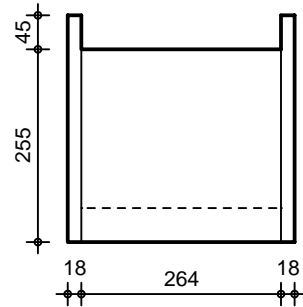
VUE LATERALE
