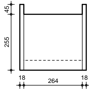
VUE LATÉRALE
