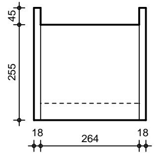
VUE LATÉRALE
