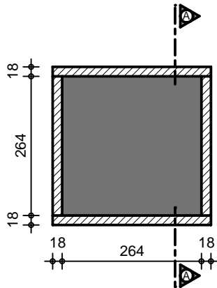
VUE EN PLAN
